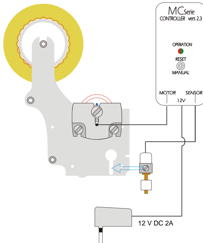
Anschluss-Schema Controller
